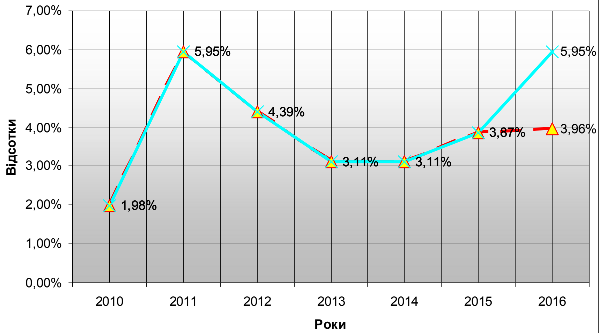
Доля альтернативного постачальника (Westinghouse) в загальному обсязі ЯП, що експлуатується на АЕС з ВВЕР-1000
